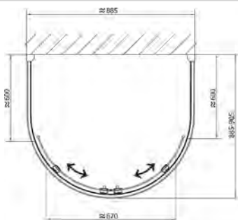
L5 - čtvercová zástěna (skládací dveře) (zde DL2715)
