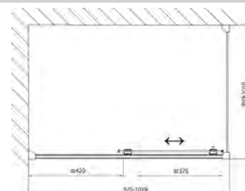
L8 - obdélníková zástěna (4-dílné dveře + boční stěna) (zde DL4215 + DL3515)
