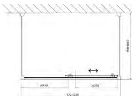
L9 - třístěnná obdélníková zástěna (4-dílné dveře+2 boční stěny) (zde DL2715+DL3515+DL1015)
