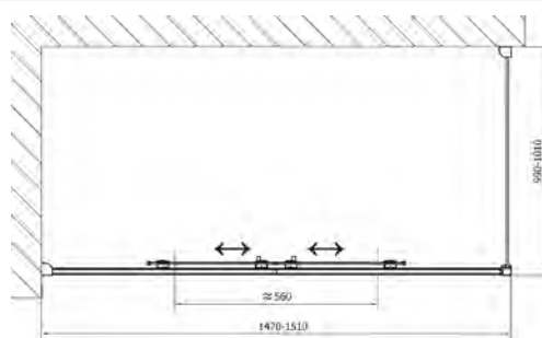
L10 - posuvné dveře do niky (zde DL1015)
