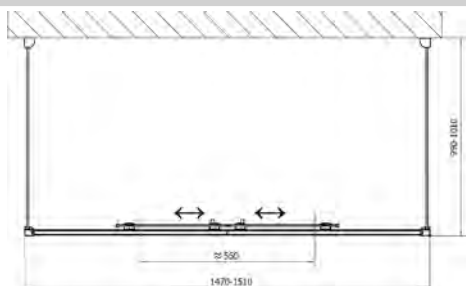
L9 - třístěnná obdélníková zástěna (4-dílné dveře+2 boční stěny) (zde DL2715+DL3515+DL1015)
