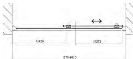
L10 - posuvné dveře do niky (zde DL1015)
