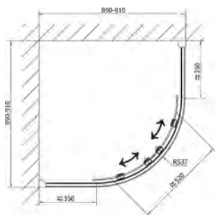
L3 - půlkruhová zástěna (zde DL3615)
